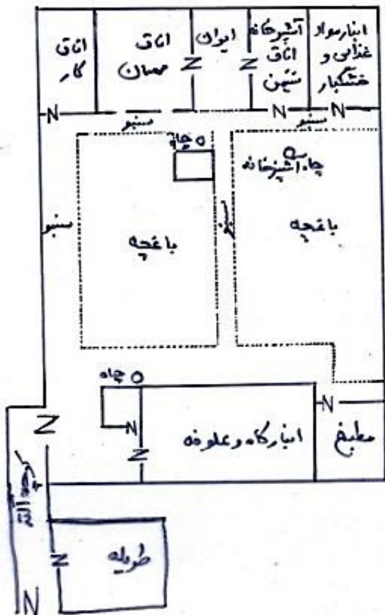
شکل ۴۵. خانه مرحوم تقی سلیمی موبد در محله قلعه همراه با راهرو و باغچه
